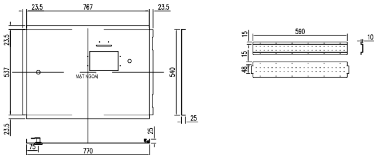
Hình 9: Thiết kế cánh cửa trước
