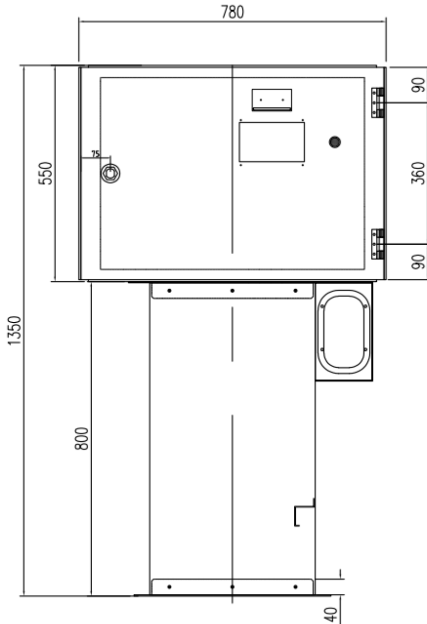
Hình 4: Kích thước mặt trước/mặt sau trụ sạc
