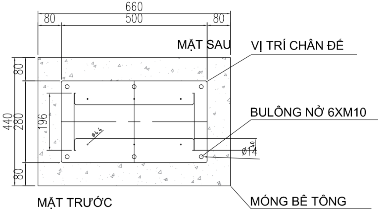
Hình 8: Kích thước chân đế lắp lên bộ móng
