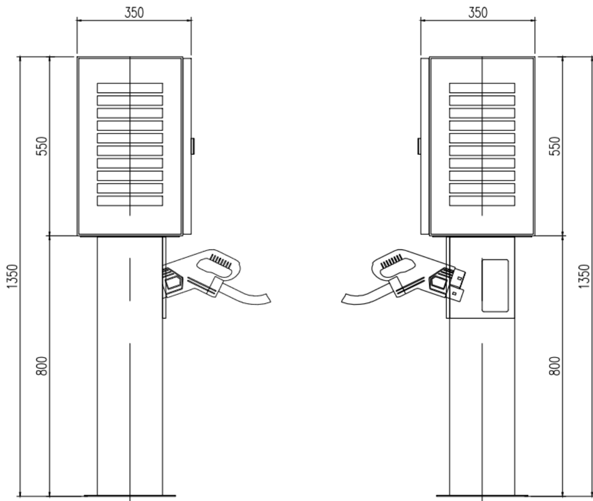
Hình 5: Kích thước hai bên trụ sạc
