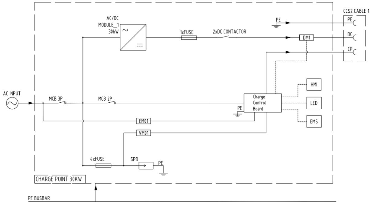
Hình 6: Sơ đồ khối của trụ sạc
